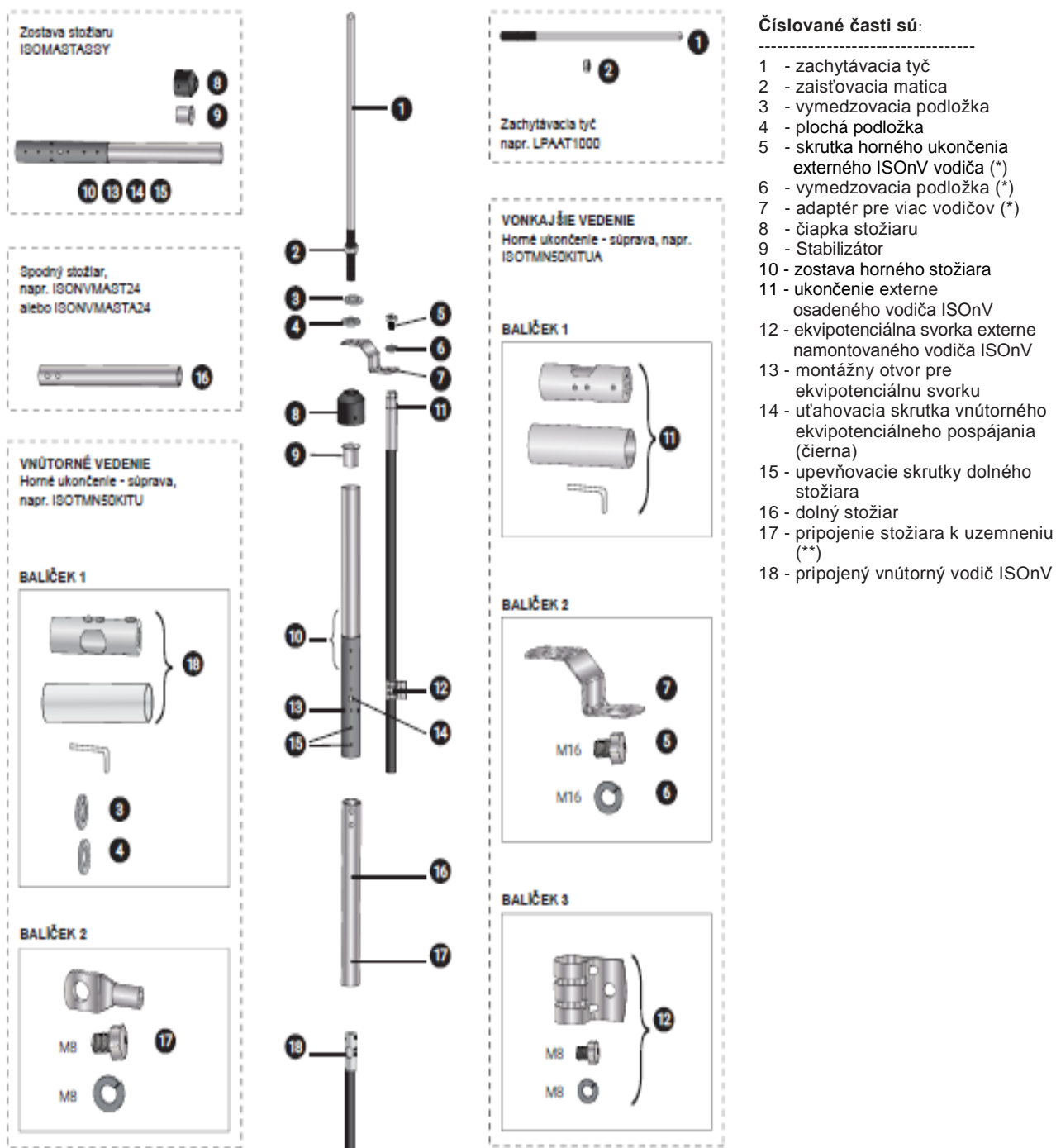
Pohľad na rozloženú zostavu stožiaru
